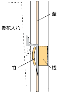
二重折釘の場合
