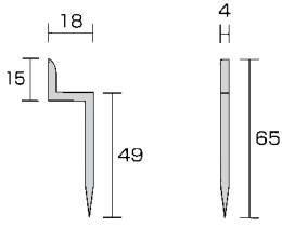
二重折釘
