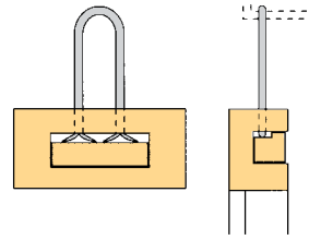
花蔓釘は足を割って埋木をして掛け雨戸の上框に仕込む
