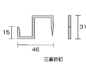
三重折釘
