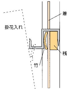
三重折釘の場合
